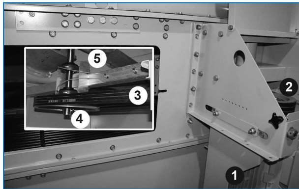
Système d'entraînement avec moteur externe
